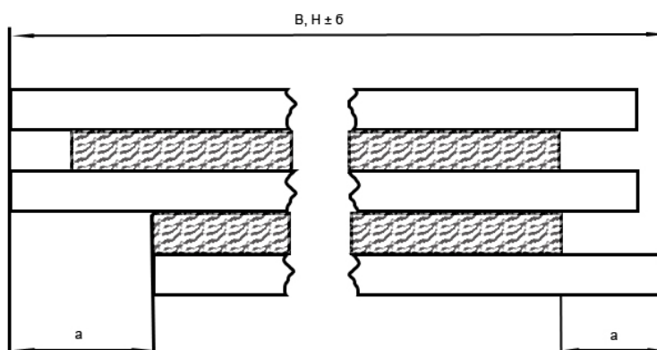
В, Н – длина и ширина многослойного стекла. а – смещение листов стекла в многослойном стекле; б – допуск на длину и ширину многослойного стекла
